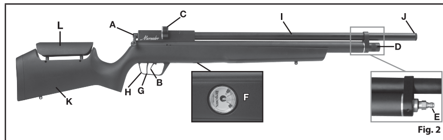
A. Bolt B. Safety C. Clip D. Protective Cap For Fill Nipple E. Fill Nipple F. Pressure Gauge G. Trigger H. Trigger Guard I. Barrel J. Muzzle K. Stock L. Stock Comb
