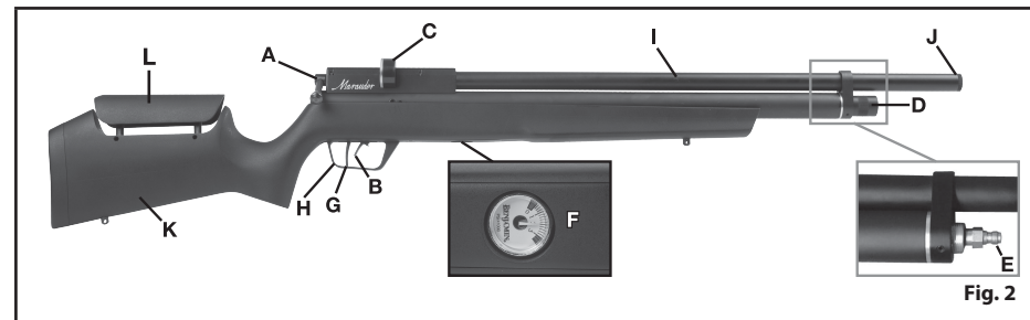
A. Cerrojo B. Seguridad C. Pinza D. Tapón protector del niple de llenado E. Niple de llenado F. Medidor de presión G. Gatillo H. Guardamonte I. Cañón J. Boca K. Culata L.
